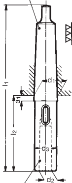
Inside taper Morse DIN 228
